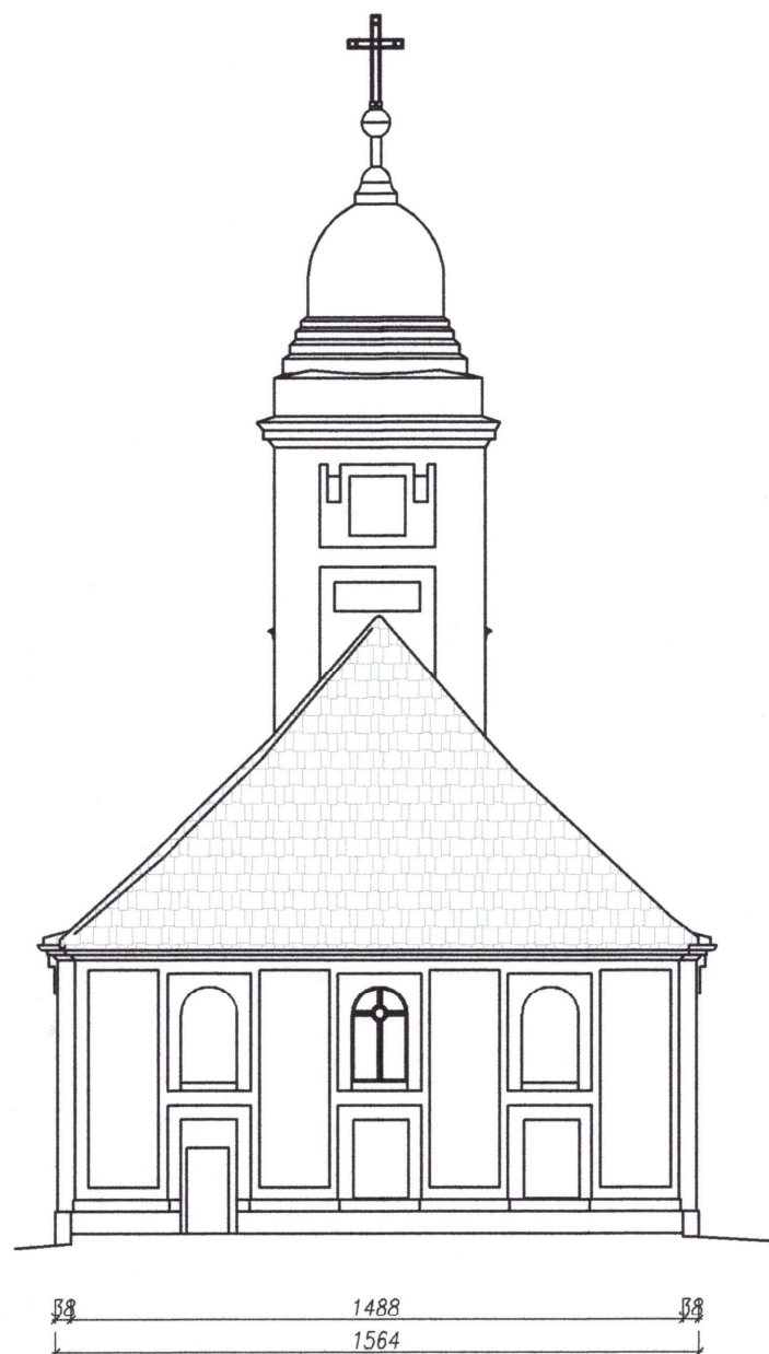
ELEWACJA PÓLNOCNIA
